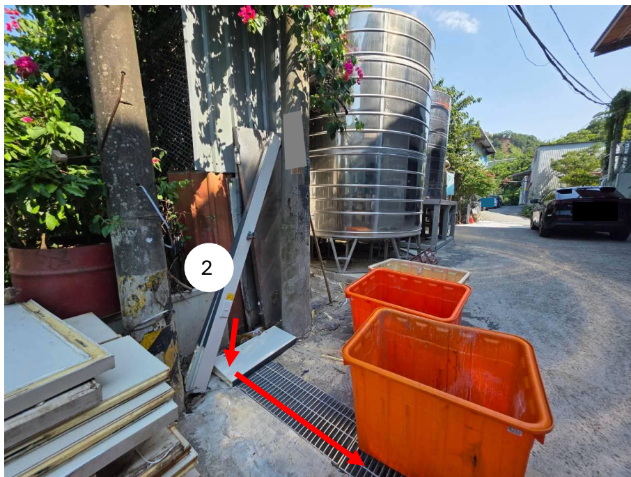
放流水流向
